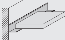
Okrajový stupňovitý profil C-SRW 25 / 15 / 8 / 15
