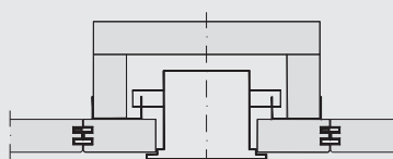
Vestavěná svítidla s protipožárním krytem
